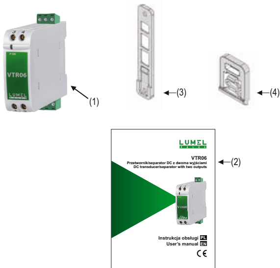
Rys. 1. Zestaw przetwornika.
